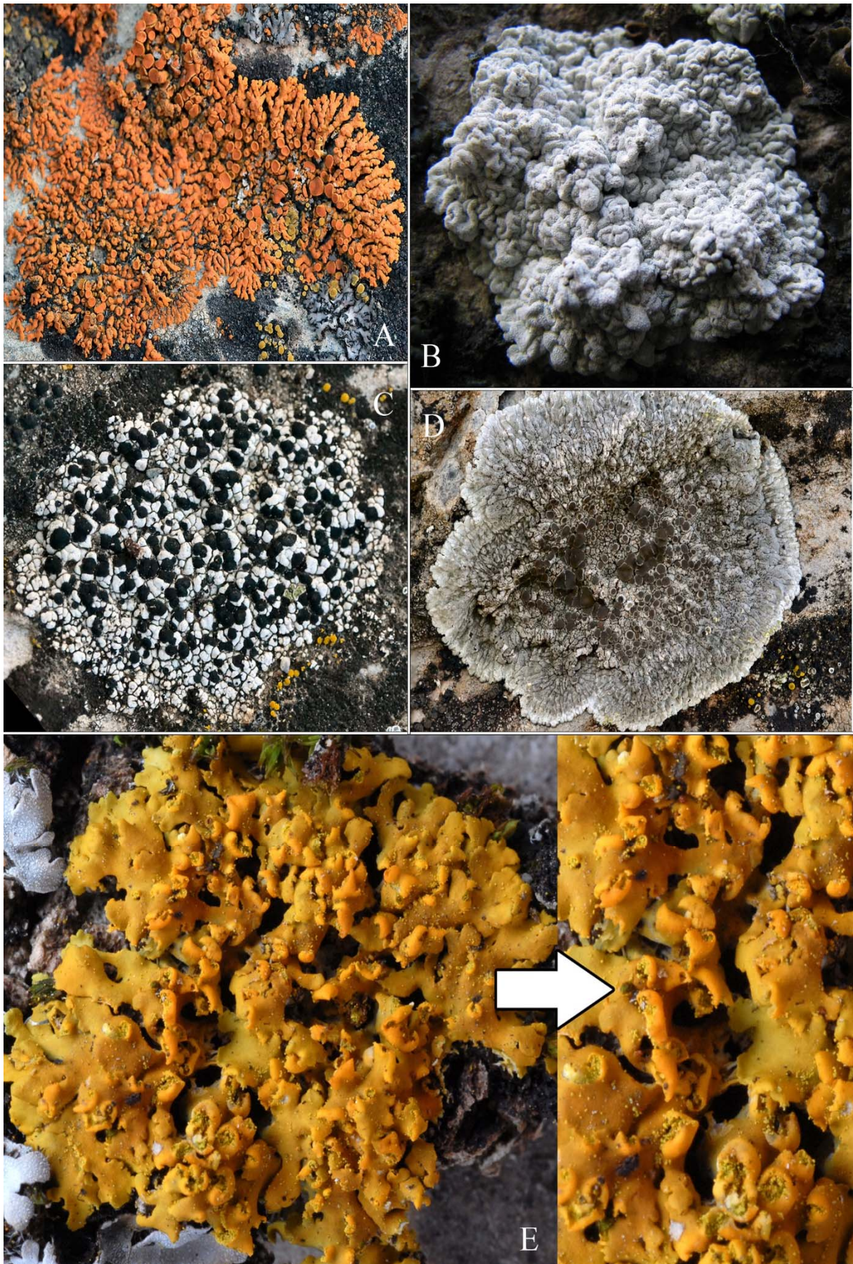
J1a. A. Xanthoria elegans (FJ). B. Toninia candida (FG). C. Lecidella carpathica (FG). D. Lobothallia radiosa (FJ). E. Xanthoria huculica et gros plan sur les soraliés marginales en forme de casque (OG).
